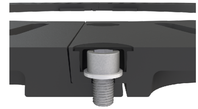
Detail Verschraubung
